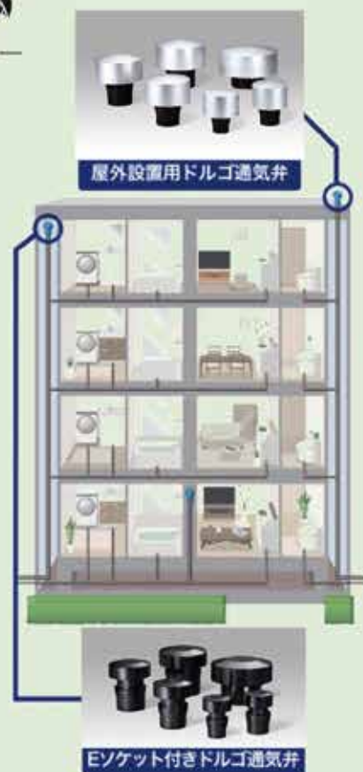
集合住宅でのドルゴ通気弁使用例
