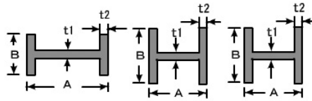
H型鋼 (細 幅)
