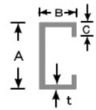
カラーC型鋼 (サビ止め付)
